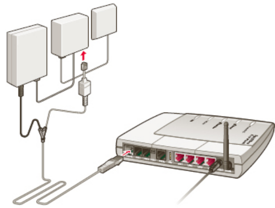
aansluiting 7170-B op NT1 (zwart) en ISDN-splitter (grijs)
